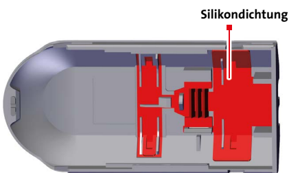
Abb. 2 Gehäuseunterteil
