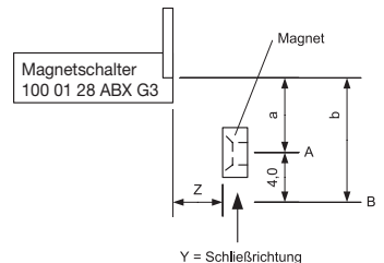
Ermittlung des idealen Montageabstandes
